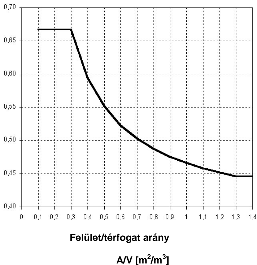
2. ábra: Az átlagos hőátbocsátási tényező követelményértékei
