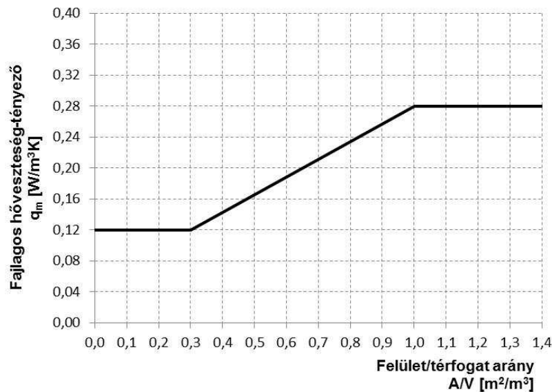
1. ábra: A fajlagos hőveszteség-tényező követelményértéke.
