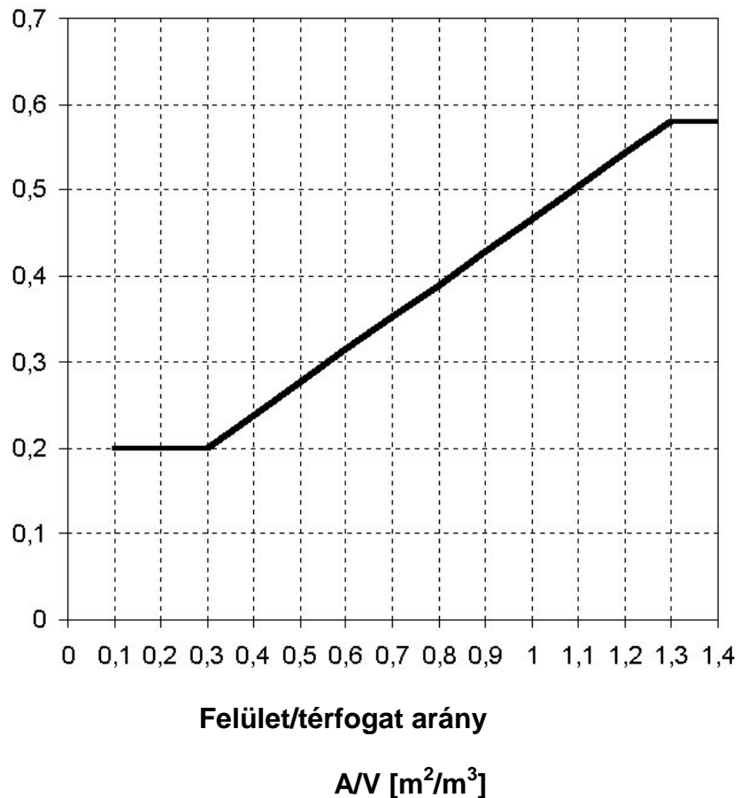
1. ábra: A fajlagos hőveszteségtényező követelményértéke
