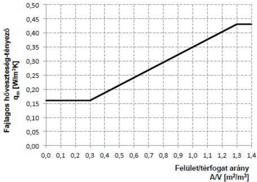
1 ábra. A fajlagos hővesztés-tényező követelményértéke
